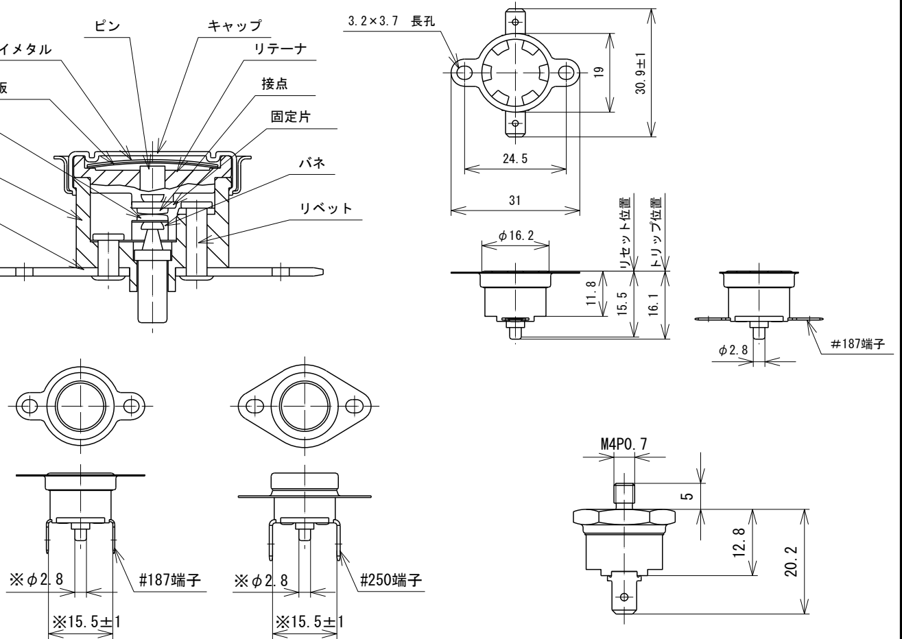
構造図(例)
